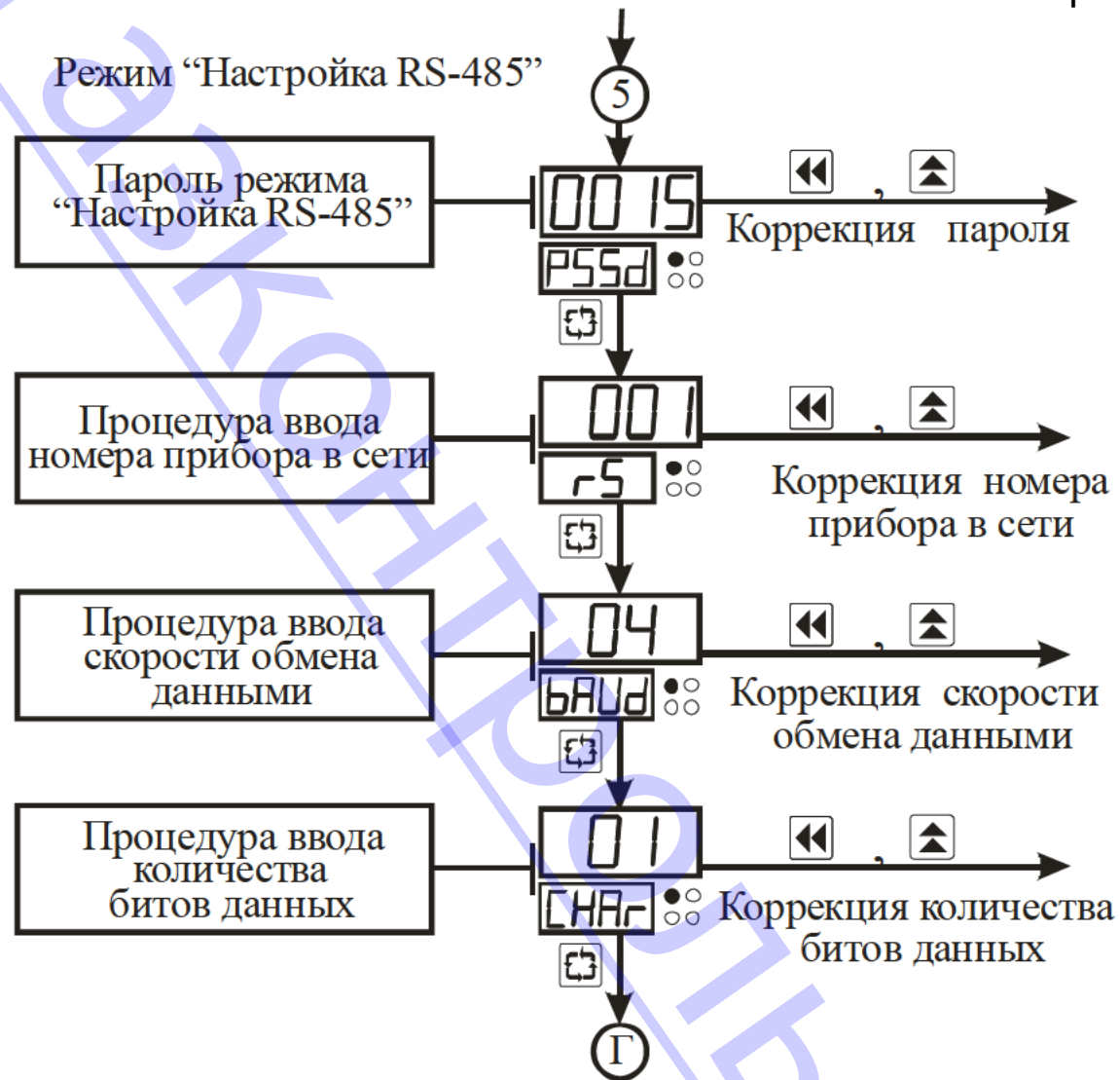
Рисунок 3.19 – Схема алгоритма работы в режиме “Настройка RS-485”
